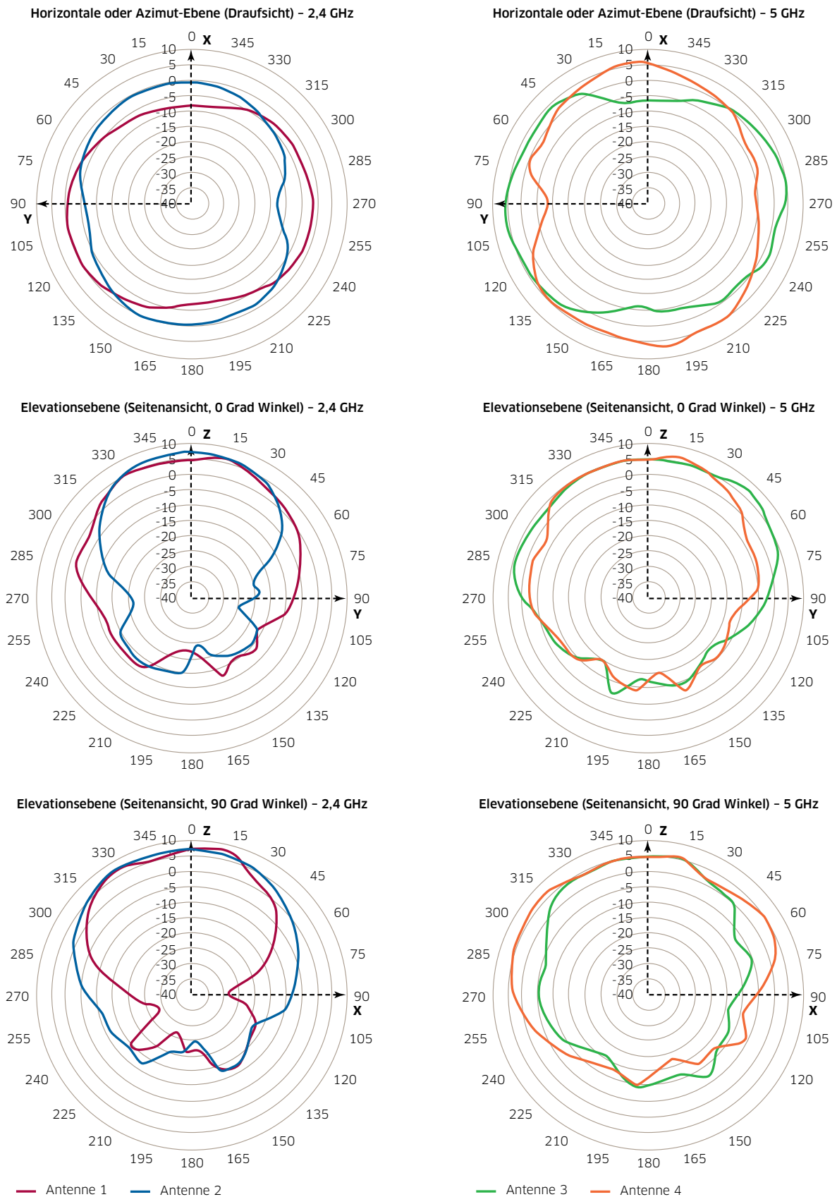
Abbildung 1. OmniAccess Stellar AP1251-Antennenmuster
